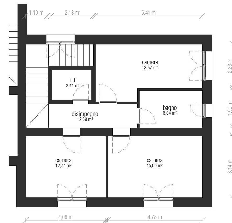
2 U402 1 : 100 piano primo edificio secondario
